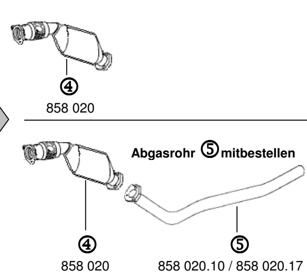
Abb.2: NACHRÜSTUNG mit Partikel-Kat
