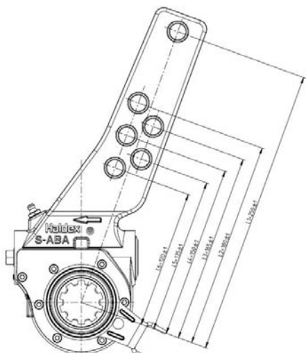
Sattelarm
