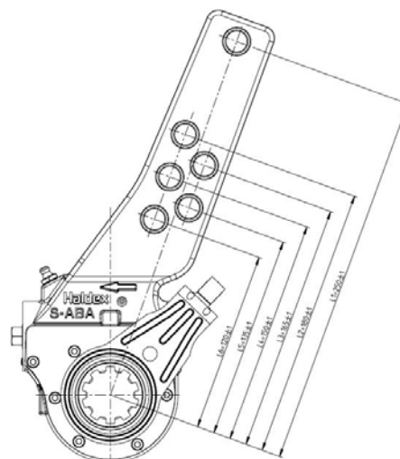
Gerollter Arm
