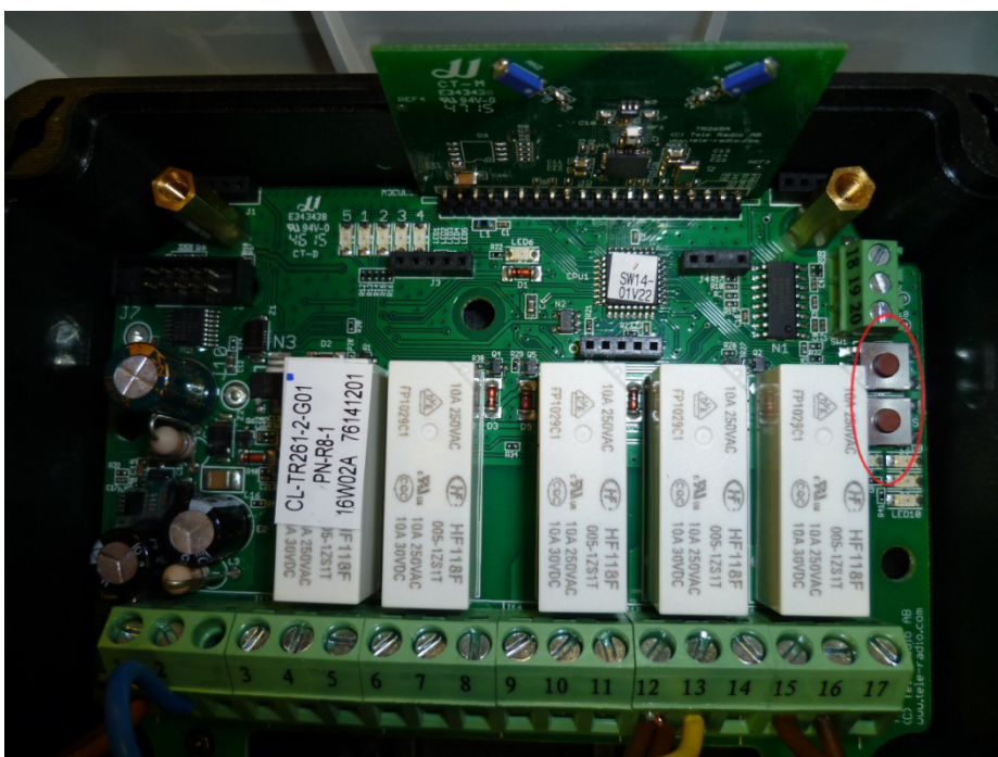
Abb. 1: Empfänger innerhalb der Steuereinheit
